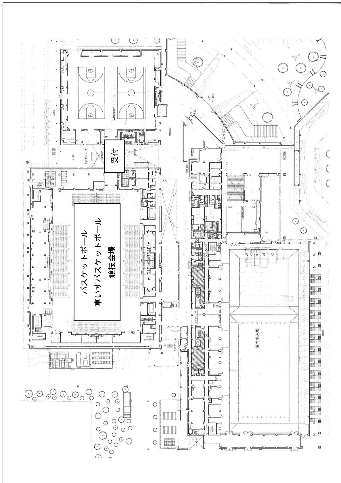
バスケットボール・車いすバスケットボール競技会場図（日環アリーナ栃木 メインアリーナ）
